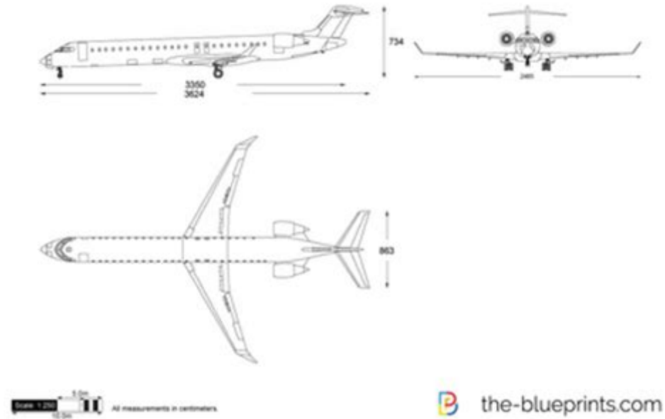
Bombardier CRJ 700-900
